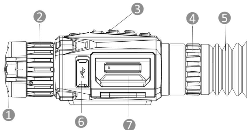
Obrázek 1-1 Vzhled I
