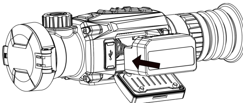
Obrázek 2-3 Vložení baterie
