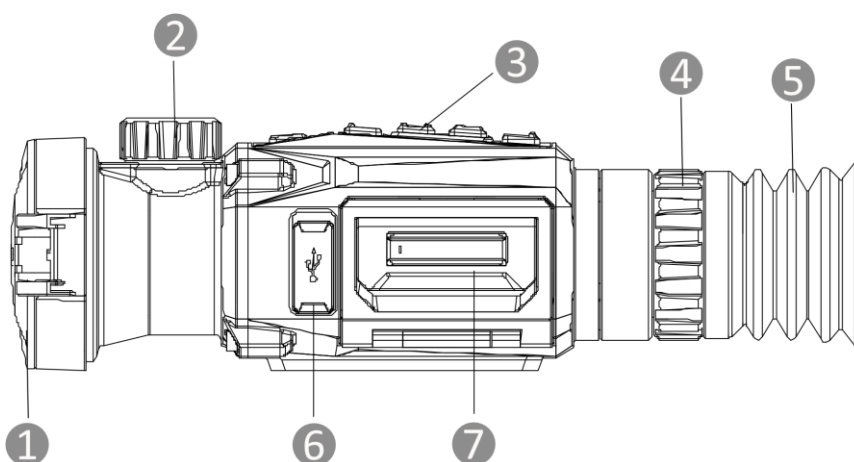
Obrázek 1-2 Vzhled II
