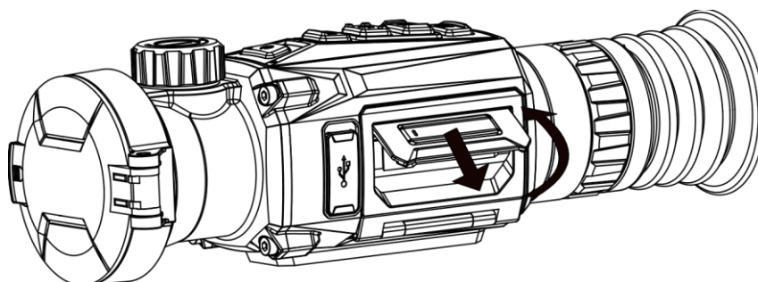
Obrázek 2-1 Vytažení krytu prostoru pro baterii
