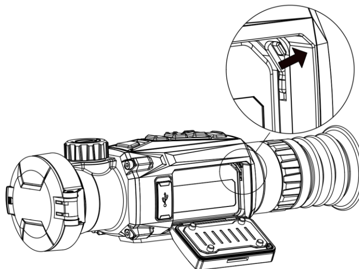
Obrázek 2-2 Odjištění západky baterie
